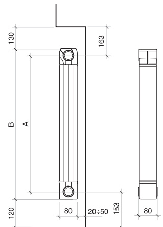
A MÉRETEK MILLIMÉTERBEN ÉRTENDŐK.
