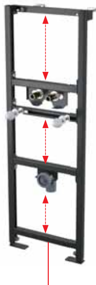
A104A/1200 szerelőkeret mosdóhoz és csaptelephez
