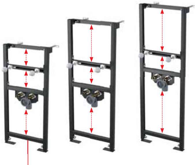
A104 850 / 1000 / 1200 szerelőkeret mosdóhoz
