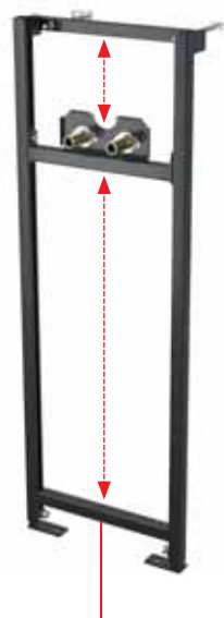
A104B/1200 szerelőkeret csaptelephez
